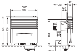
Einbauabmessungen S 3004
